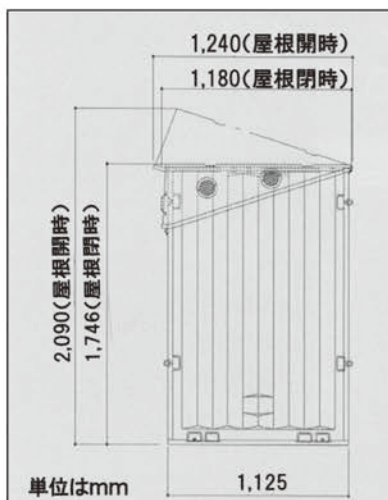
■寸法図
