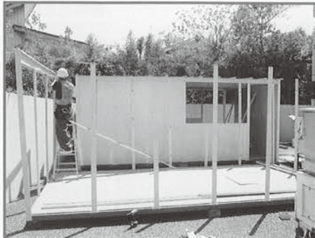
妻側1.5間までが片流れ屋根となります。
