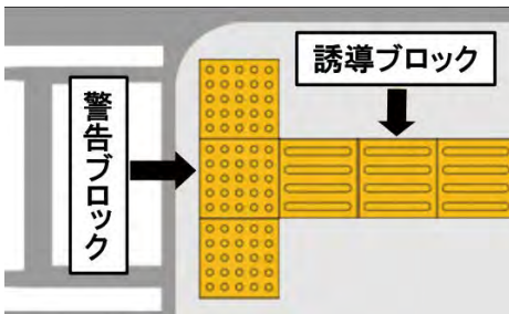
■誘導・警告点字ブロックの設置例です。
