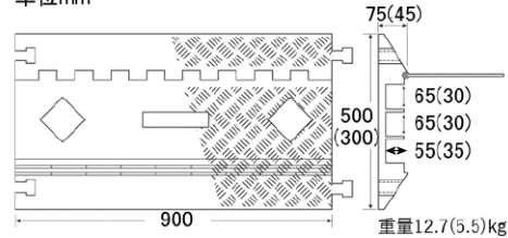
■( )はミディアム収納タイプの数値です。
