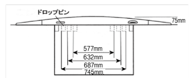
■エンドプレート
