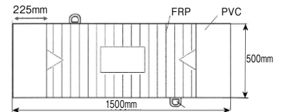
■かいさくロードプレート
