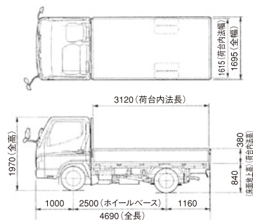
2トン平レギュラー
