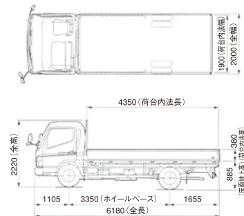
2トン平ワイドロング
