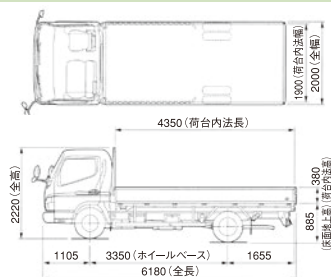
2トン平ワイドロングパワーゲート付
