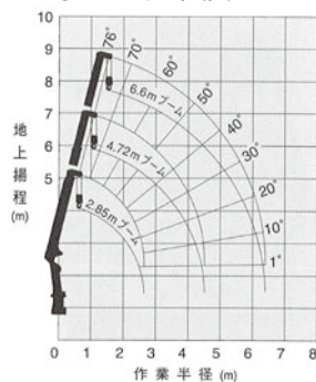
●2tユニック性能表
