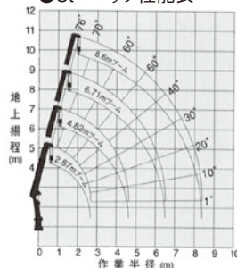
●4tユニック性能表
