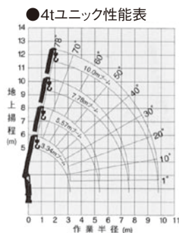
●4tユニック性能表
