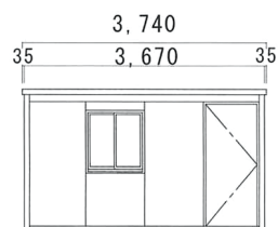
桁側立面図
