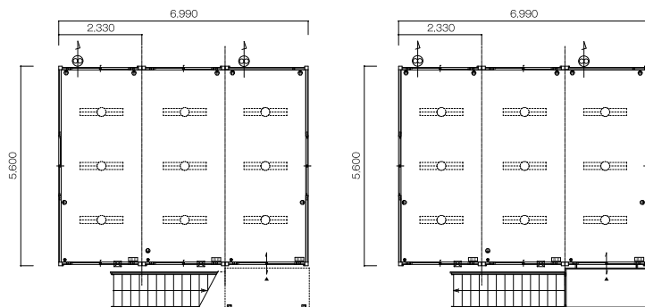
施工例：3連棟2階建て
