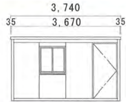
桁側立面図
