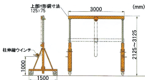
■移動はキャスタで楽々
