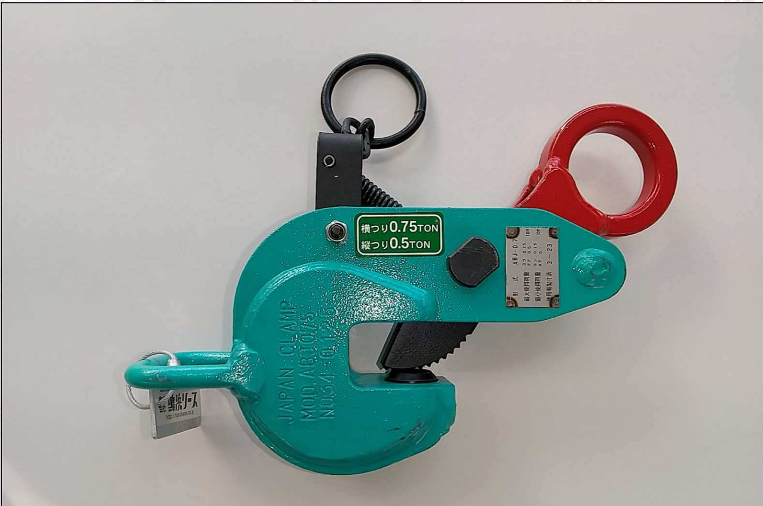
【寸法表】
