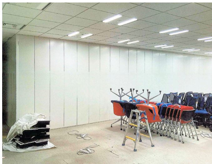
▶ 会議室
