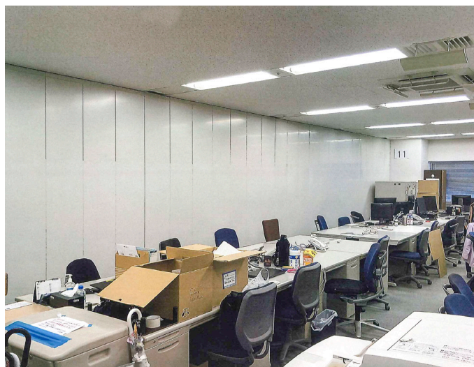
▶ オフィス
