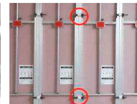
設置完了
