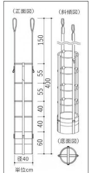
■寸法 吊れるくんロング
