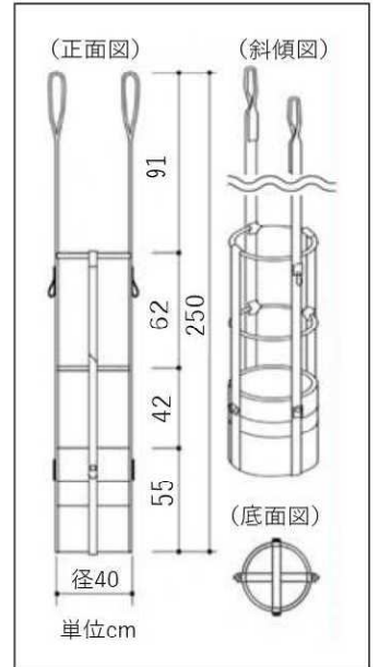
■寸法 吊れるくんレギュラー
