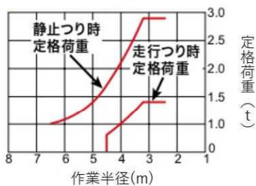
■移動式クレーン定格荷重曲線
