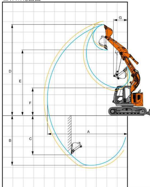
■作業範囲図
