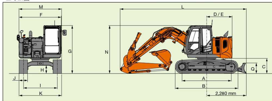
■寸法
