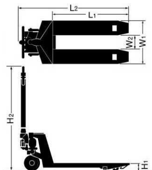
■ 寸法図
