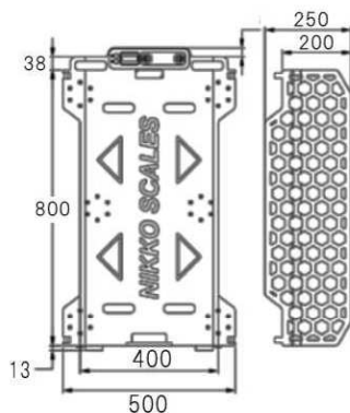
■1枚で最大20tまで計測可能。走行しながら計量も可能。
